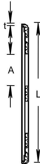
DOUBLE RECEPTACLE, TYPE DRC, 077740
