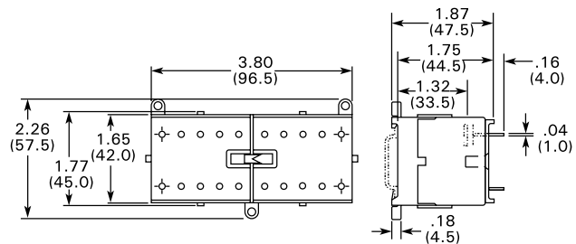
Contadores mecánicamente interbloqueados CD52BNP con terminales de pin de soldadura
