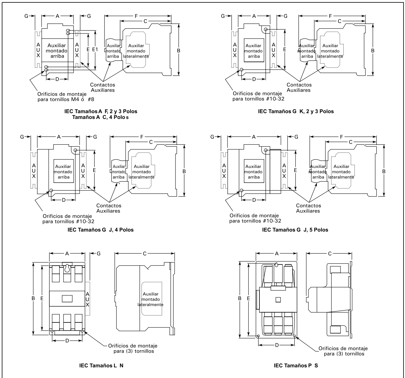
Figura 20-43. Dimensiones Aproximadas
