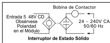
Figura 20-42. Aplicación típica
