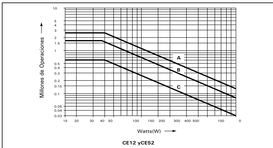
Figura 20-17. Curvas de carga-vida CD
