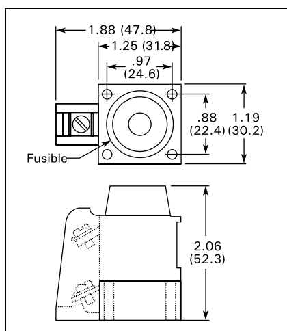
Figura 20-41. Dimensiones Aproximadas
