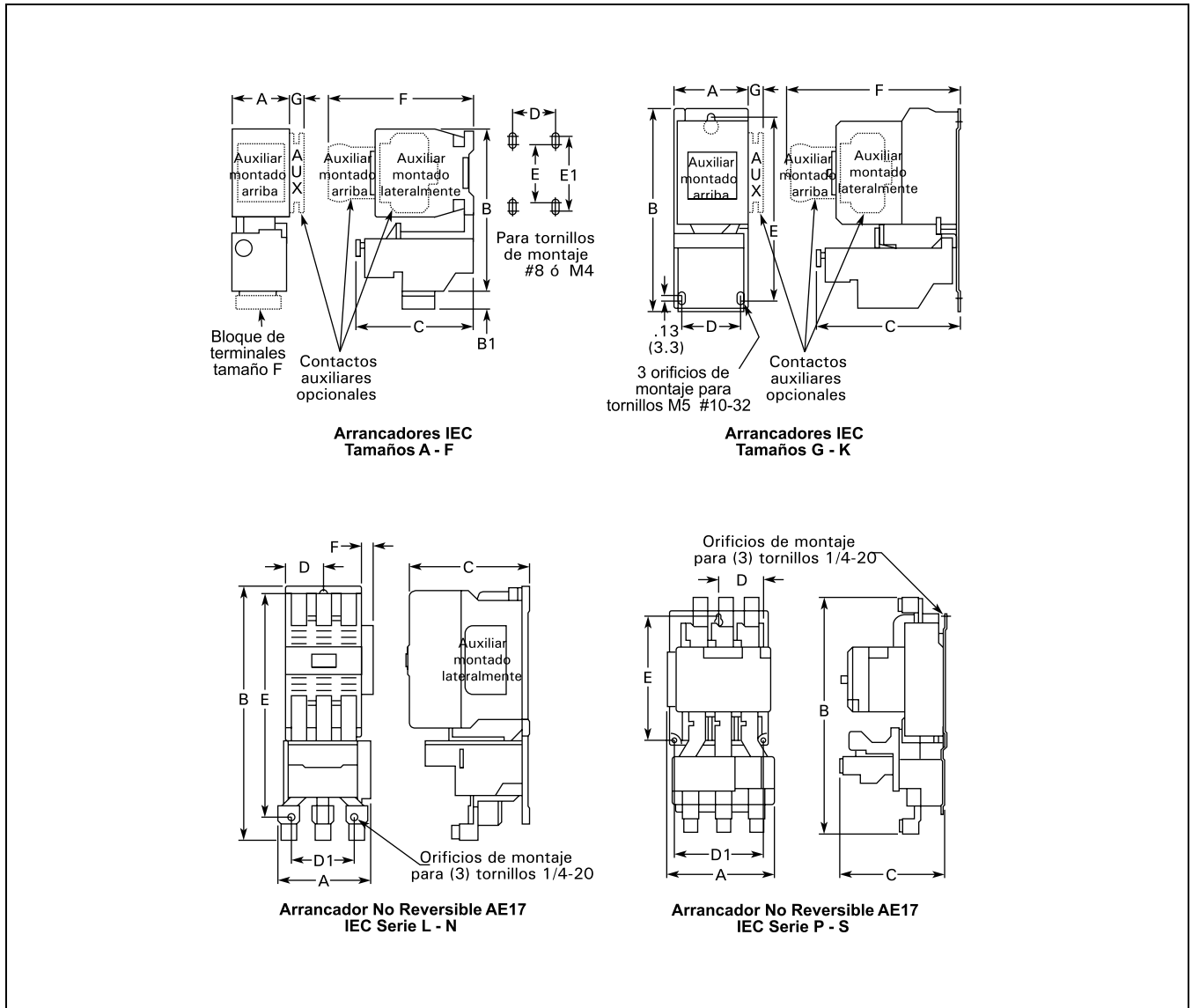
Figura 20-46. Dimensiones Aproximadas
