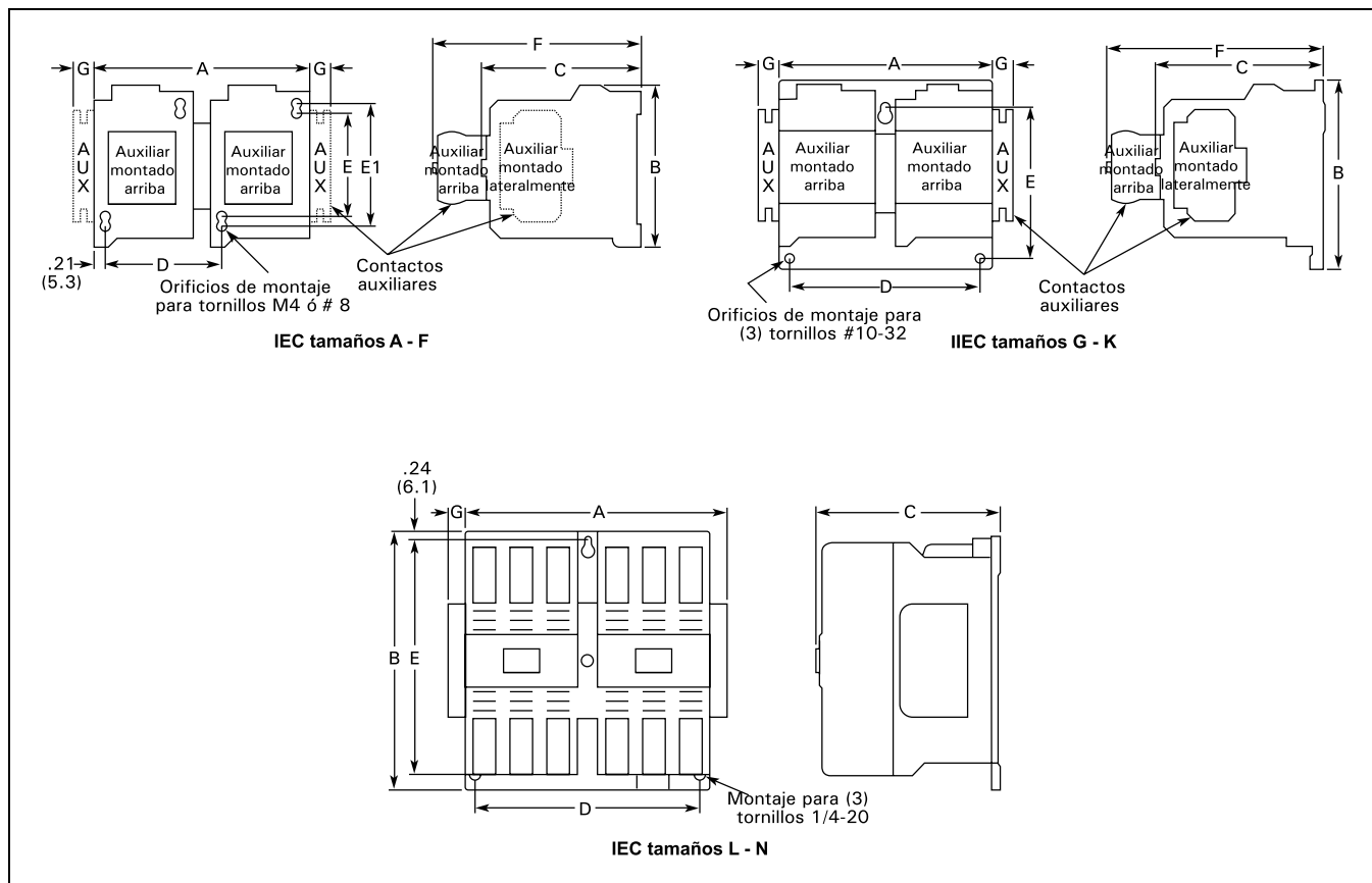
Figura 20-45. Dimensiones Aproximadas
