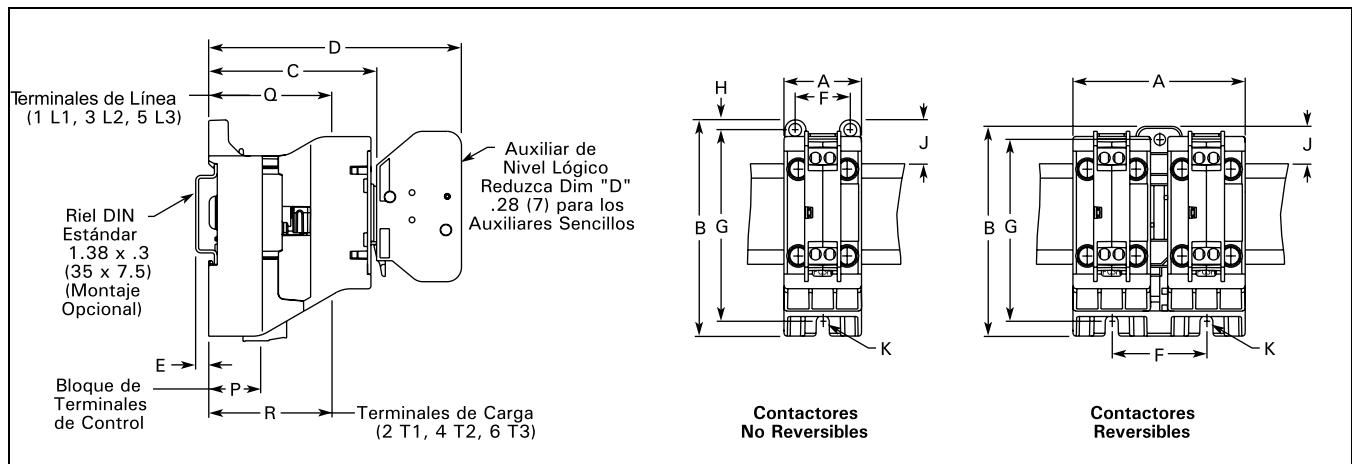
Figura 20-6. Dimensiones Aproximadas — Pulgadas (mm)
