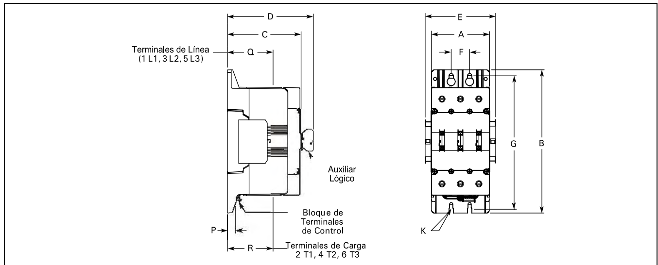
Figura 20-10. Dimensiones Aproximadas en Pulgadas (mm)
