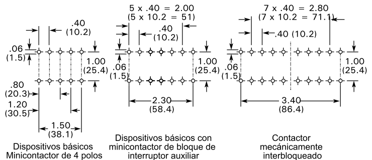
Contadores mecánicamente interbloqueados CE52BN (C B P) con terminales de placa de presión de tornillo, conexión rápida y pin de soldadura
