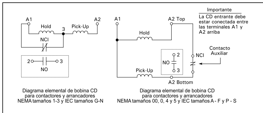
Figura 20-38. Diagramas elementales
