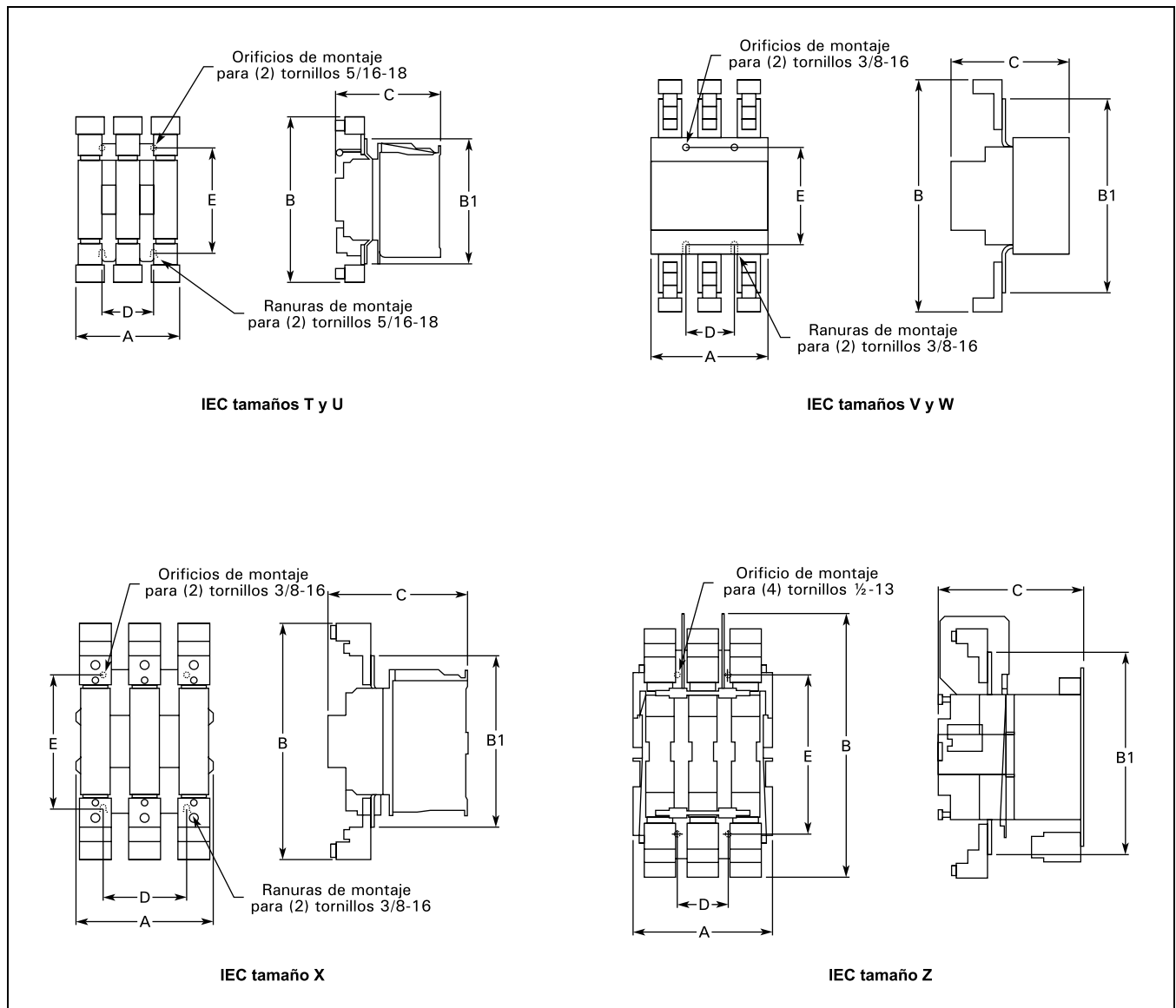
Figura 20-44. Dimensiones Aproximadas
