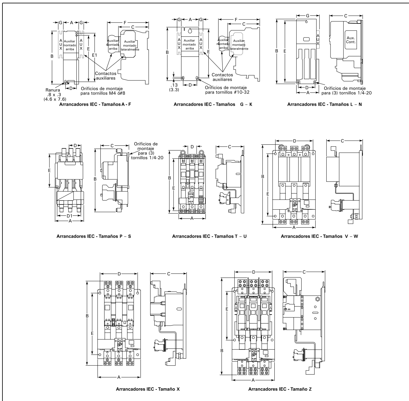
Figura 20-49. Dimensiones Aproximadas
