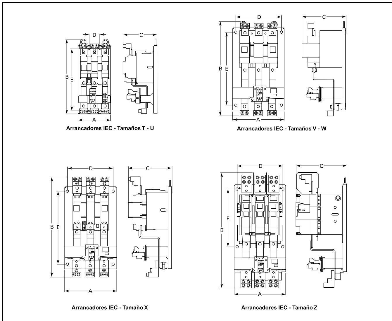
Figura 20-47. Dimensiones Aproximadas
