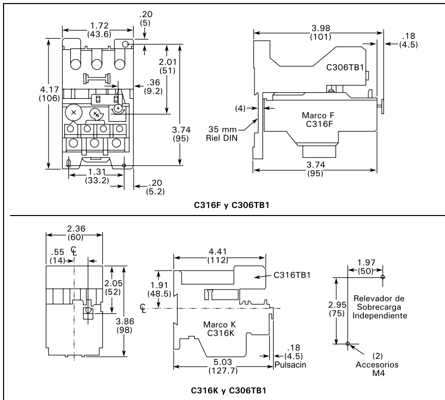
Figura 20-31. Relevadores de sobrecarga independientes — Dimensiones Aproximadas en Pulgadas (mm)
