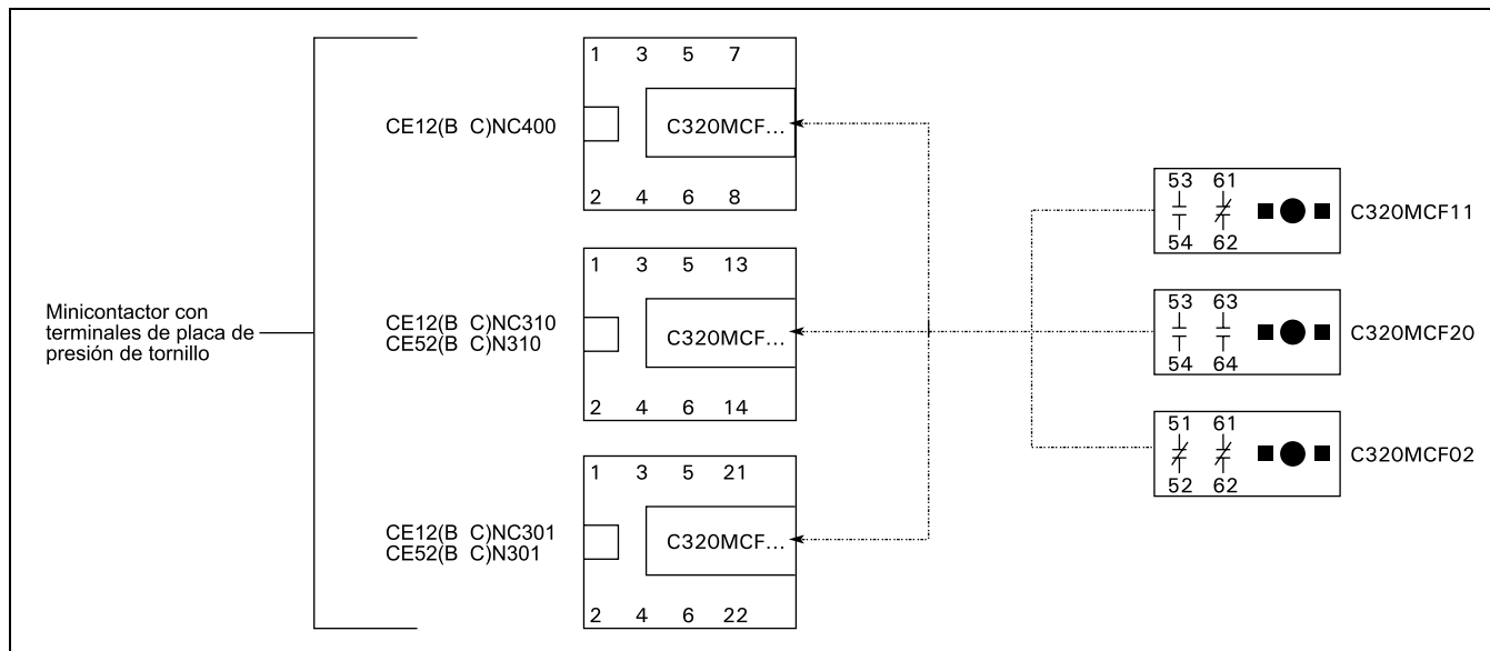
Figura 20-23. Marcas de terminales para bloques de contactos auxiliares montados en la parte frontal
