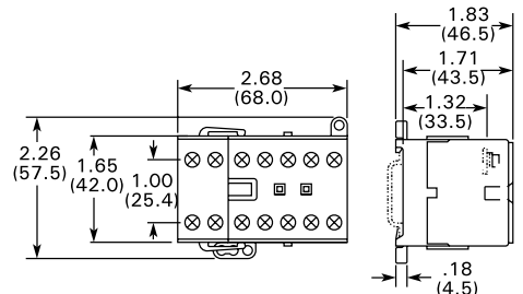
Minicontactor CE12 (B ó C) (Operado con CA y CD) con bloque de contactos auxiliares C320 (montado lateralmente) para terminales de placa de presión de tornillo y de conexión rápida
