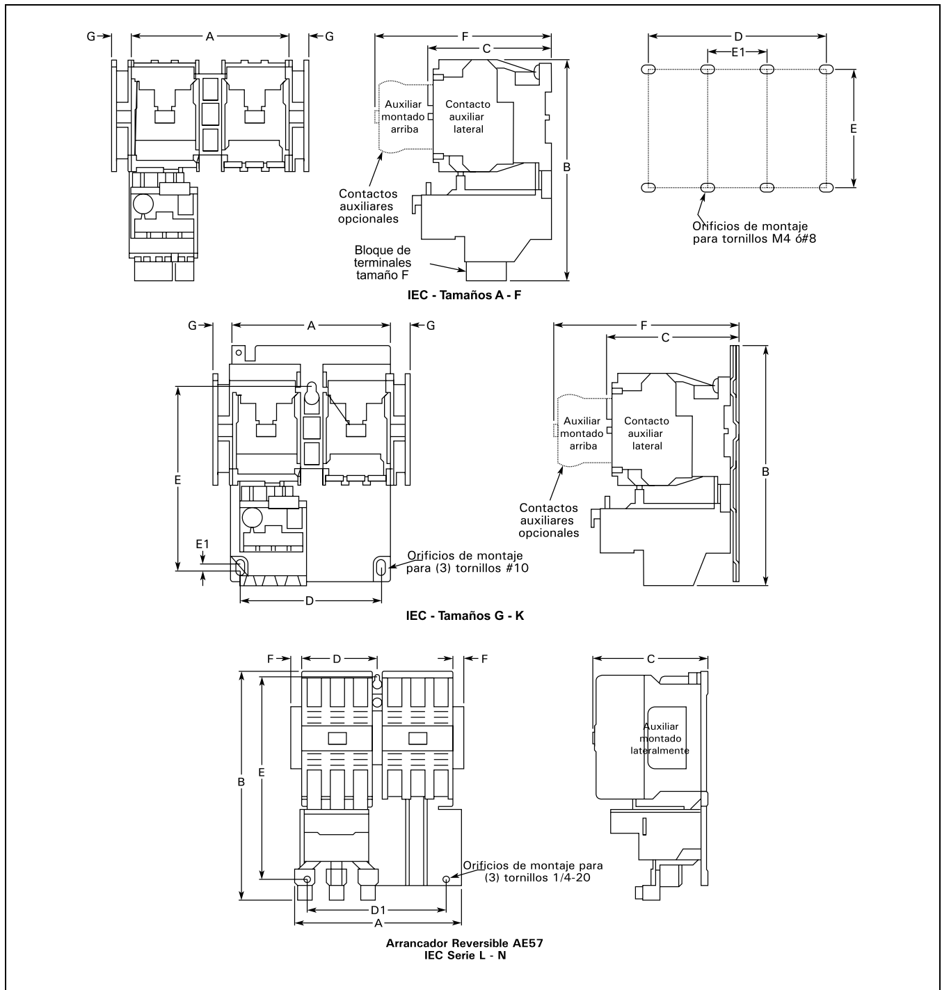
Figura 20-48. Dimensiones Aproximadas
