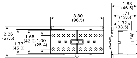
Contadores mecánicamente interbloqueados CE52BNC con terminales de placa de presión de tornillo y conexión rápida
