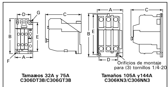
Figura 20-35. Dimensiones Aproximadas
