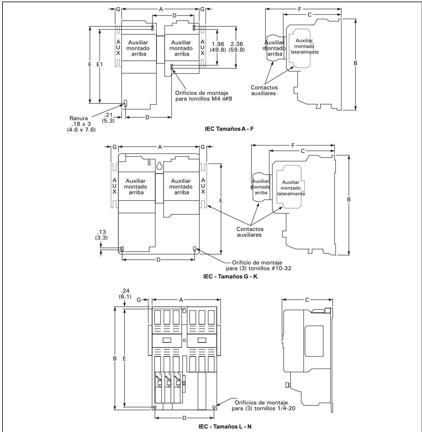
Figura 20-50. Dimensiones Aproximadas
