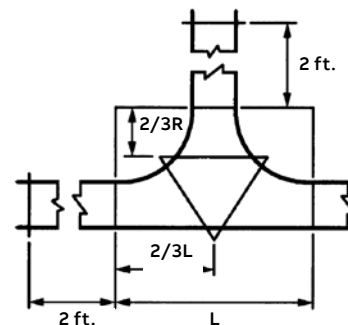
Horizontal tee
