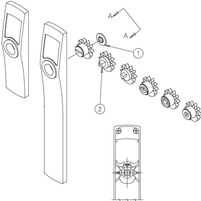
DETAIL A-A
