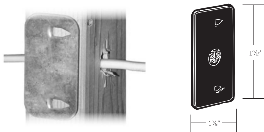
Cable Protector
