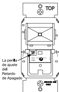
Fig 6: Ajuste de la demora de tiempo
