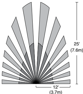
Fig 1: Patr n de cobertura del sensor
