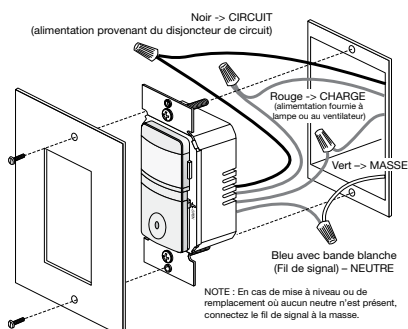
Fig. 4: Orientation du détecteur, branchement des fils et montage de boîtier mural
