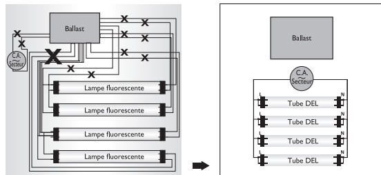
Convertir un luminaire à 3 ou 4 lampes et 1 ballast
