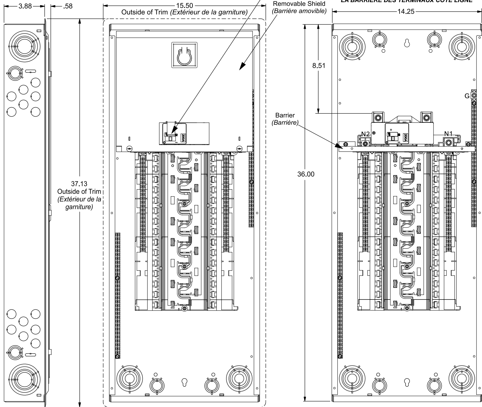
Trim Assembly represented by dashed lines (Assemblage de la garniture représentée par des lignes pointillées)
