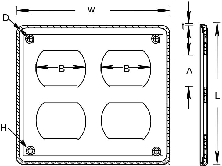
DOUBLE RECEPTACLE, TYPE DRC, 077740
