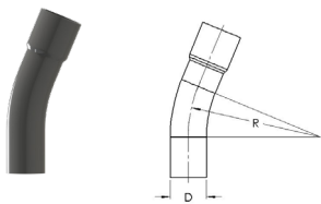
22½° Bell End
